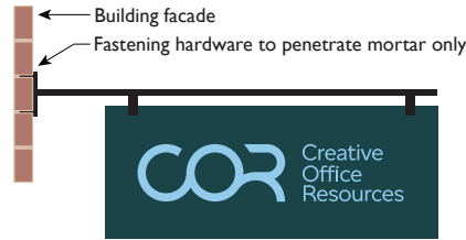
SIGN DETAIL SCALE: 1" = 1'-0"
